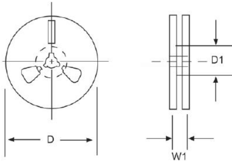
Fig 4. Reel dimensions
